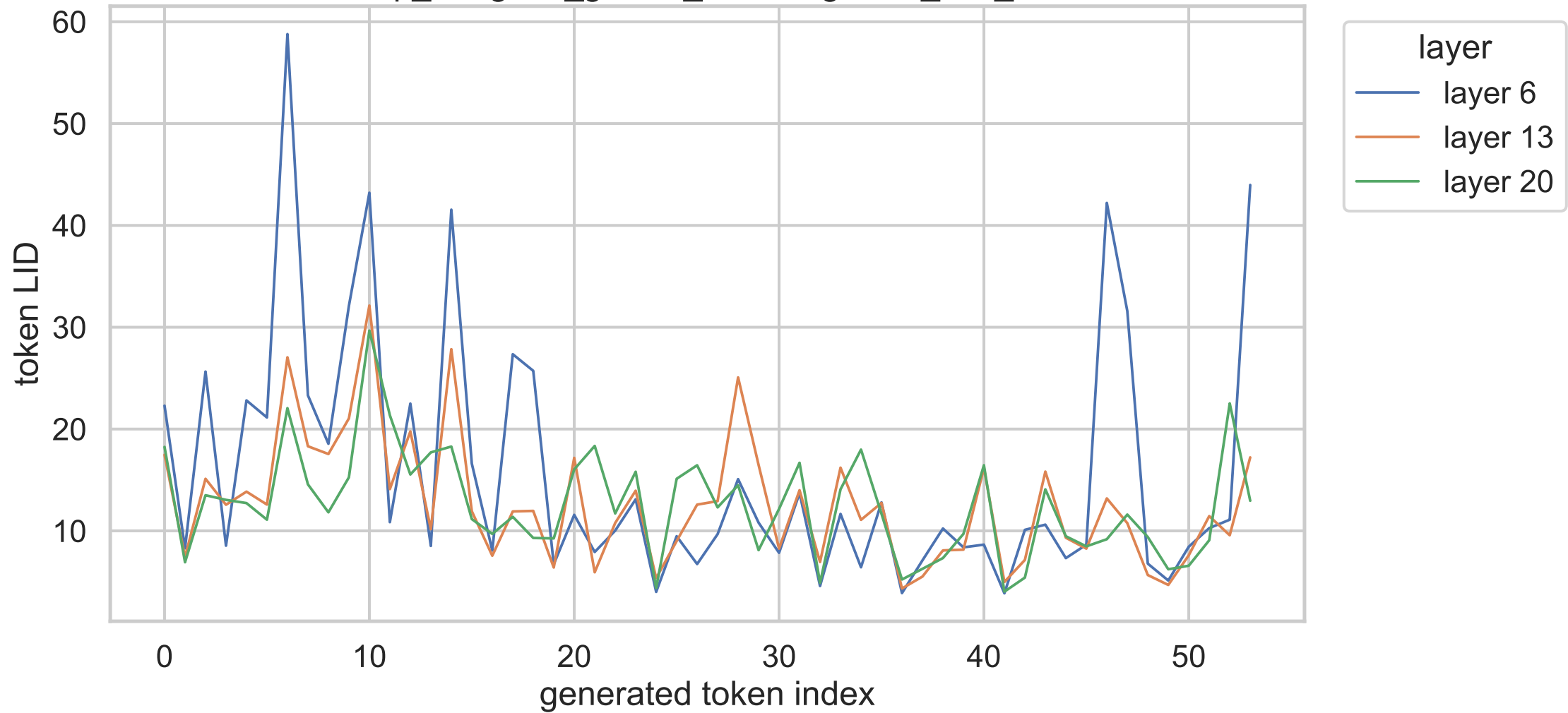
14B exp_a regular_gsm8k_nothink gsm8k_test_000345
