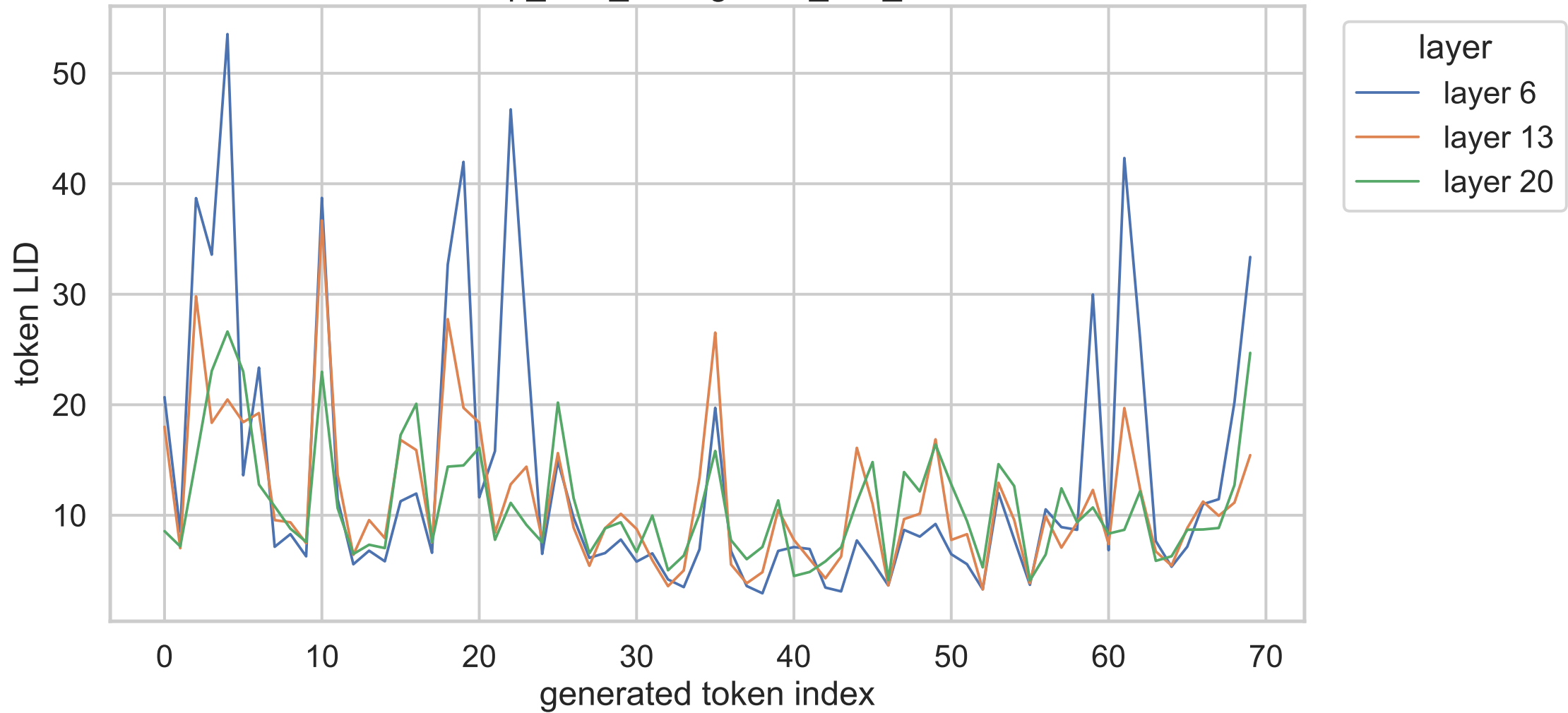
14B exp_c no_think gsm8k_test_001165
