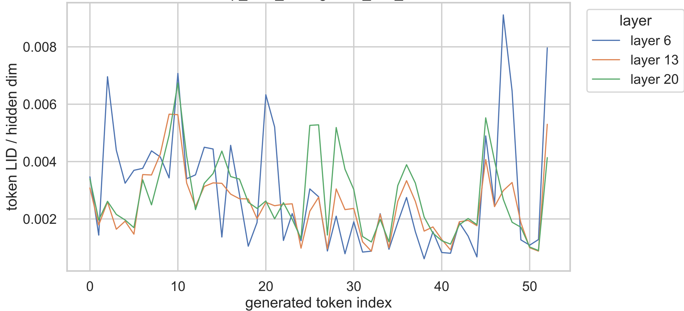
32B exp_c no_think gsm8k_test_000956
