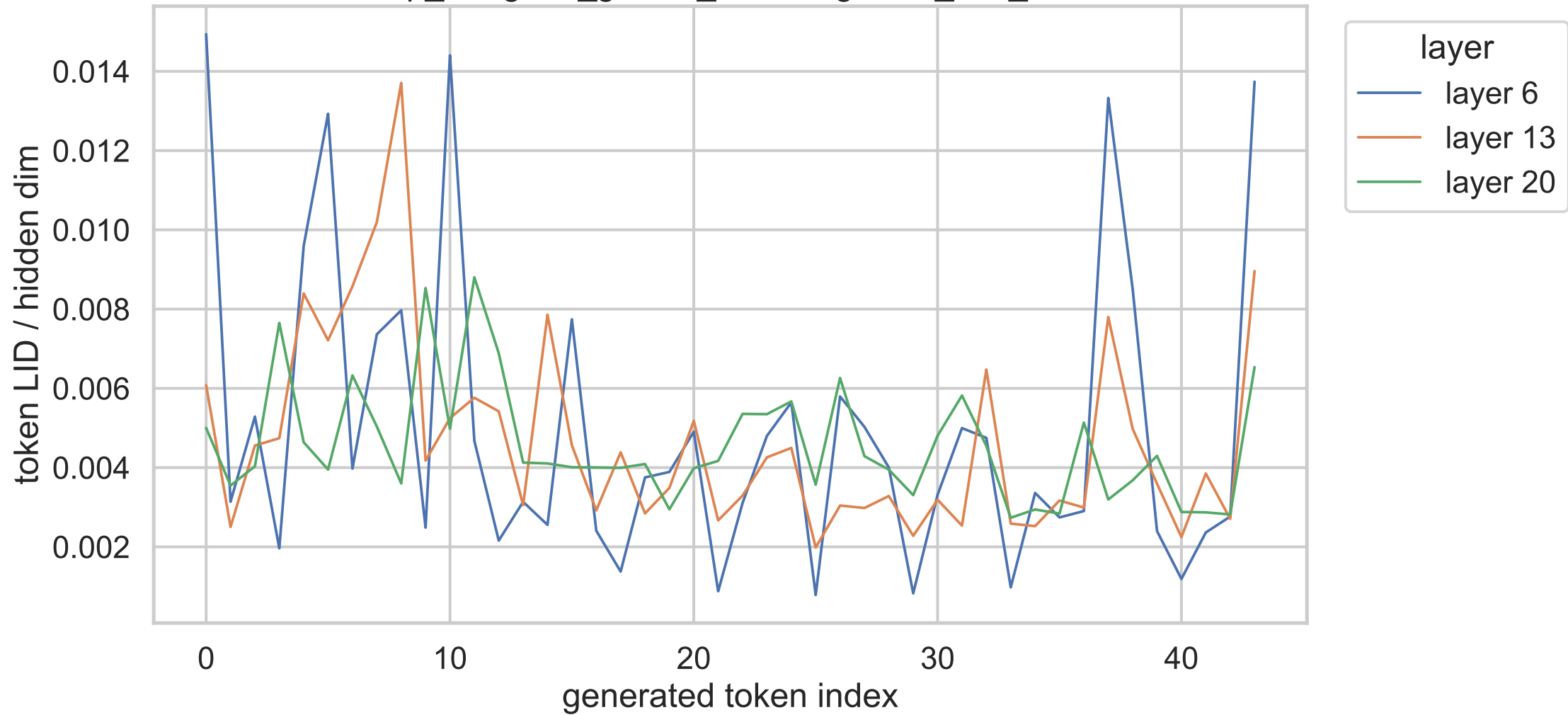
4B exp_a regular_gsm8k_nothink gsm8k_test_000850
