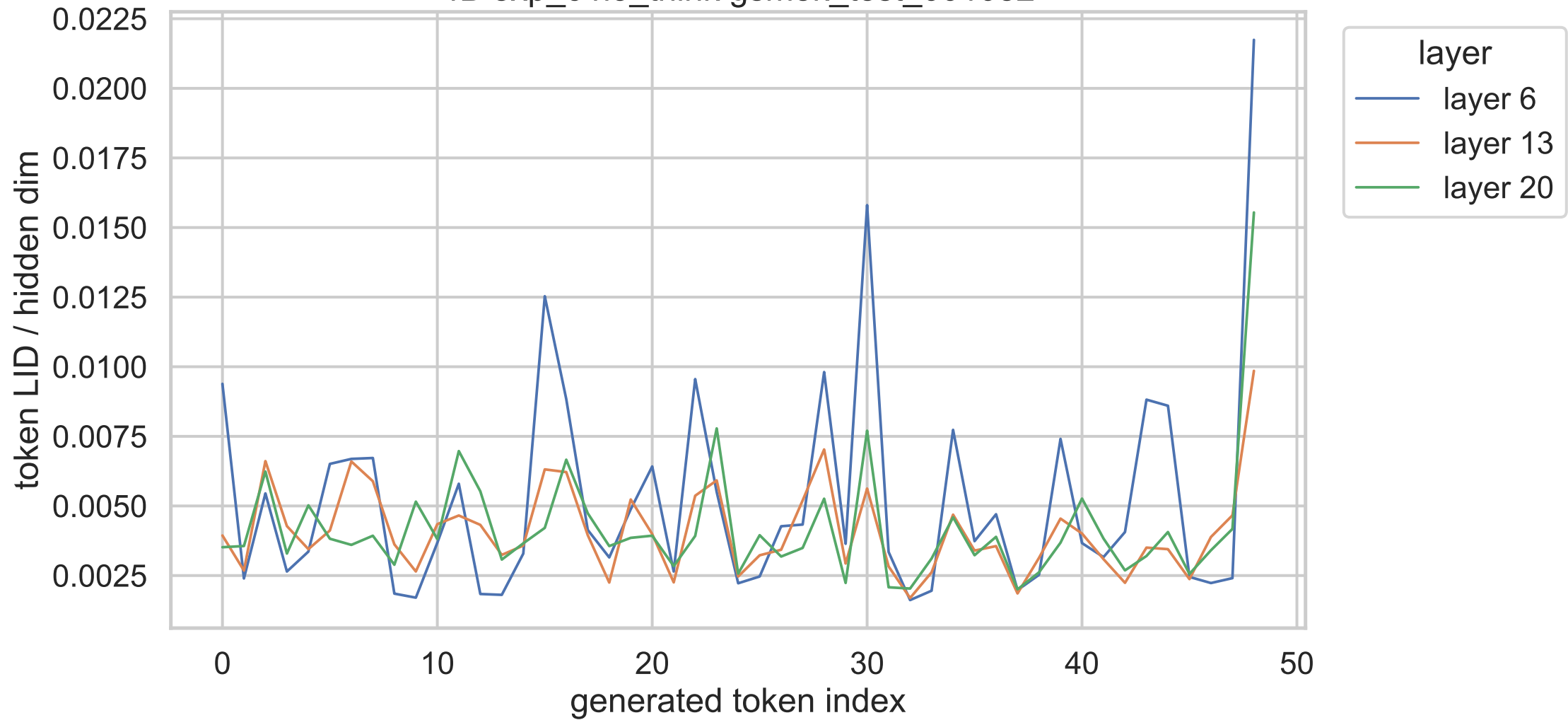
4B exp_c no_think gsm8k_test_001082
