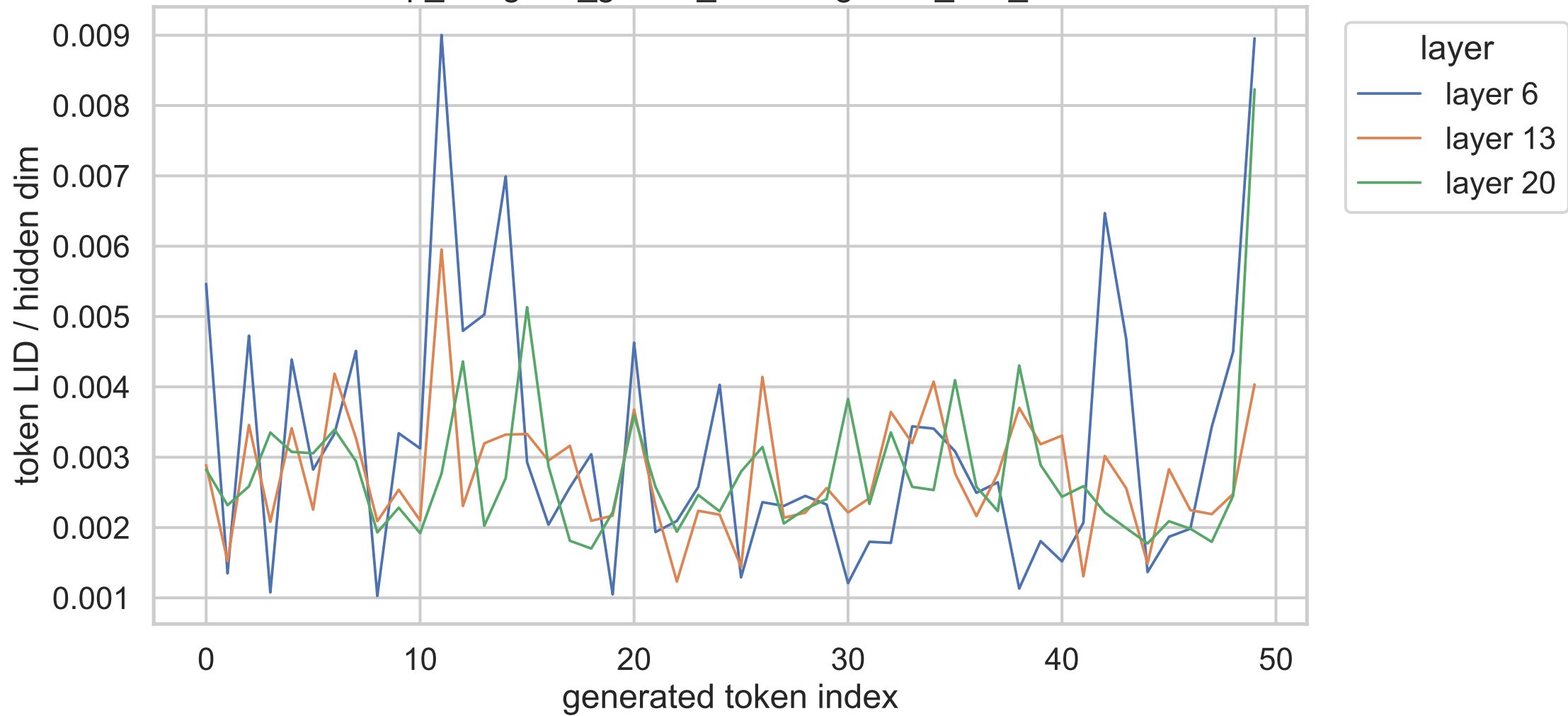
8B exp_a regular_gsm8k_nothink gsm8k_test_000345
