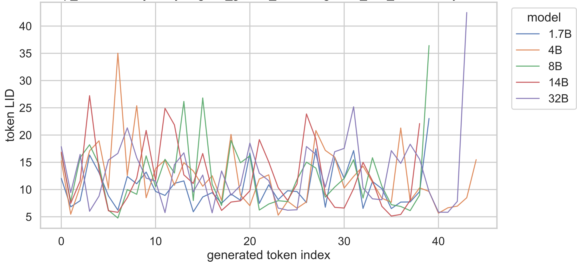
exp_a shared trajectory, regular_gsm8k_nothink, gsm8k_test_000180, layer 13
