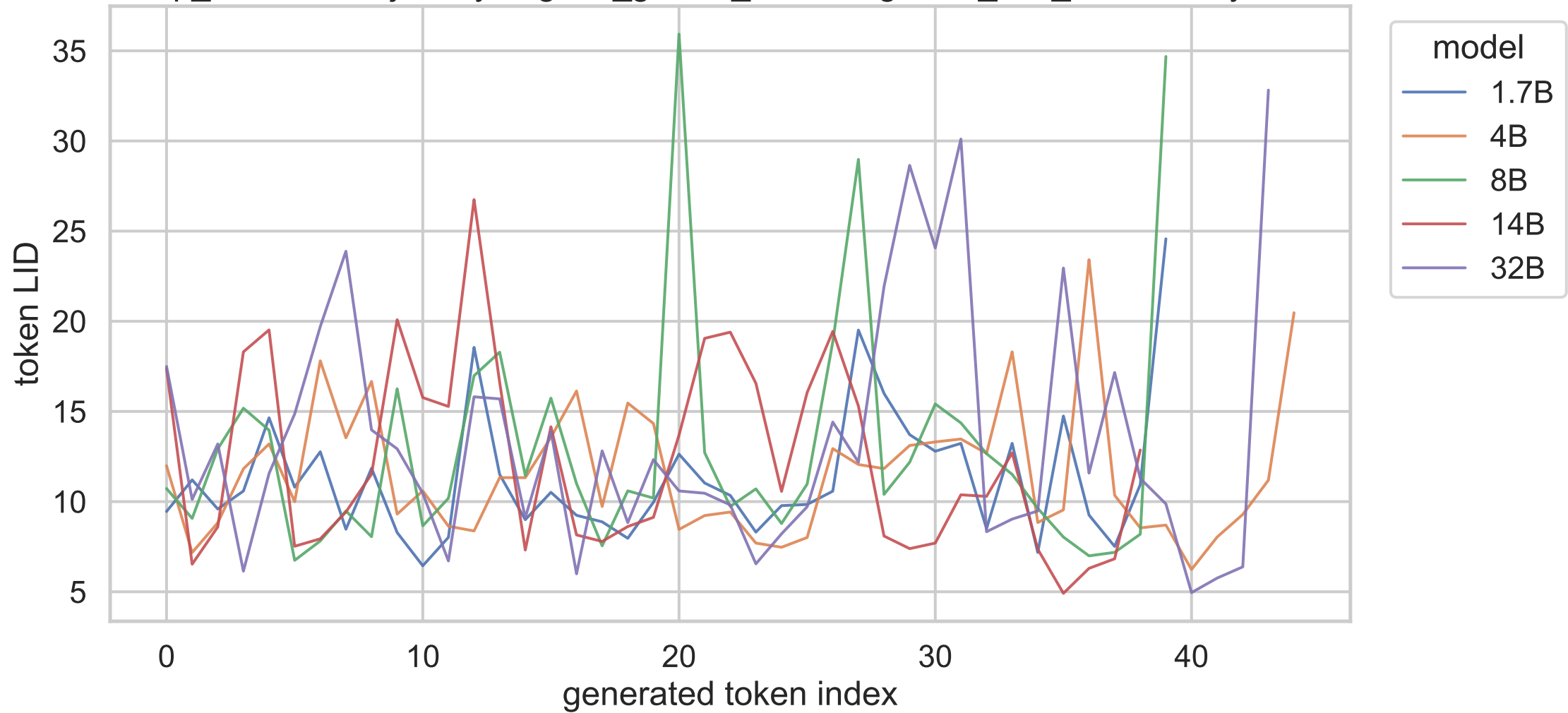
exp_a shared trajectory, regular_gsm8k_nothink, gsm8k_test_000180, layer 20
