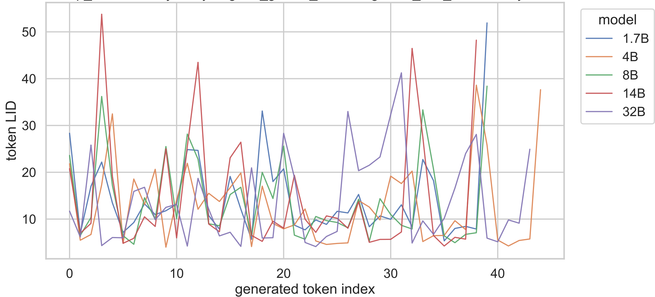
exp_a shared trajectory, regular_gsm8k_nothink, gsm8k_test_000180, layer 6
