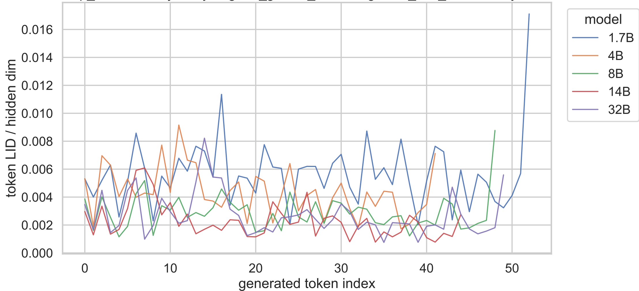
exp_a shared trajectory, regular_gsm8k_nothink, gsm8k_test_000135, layer 13
