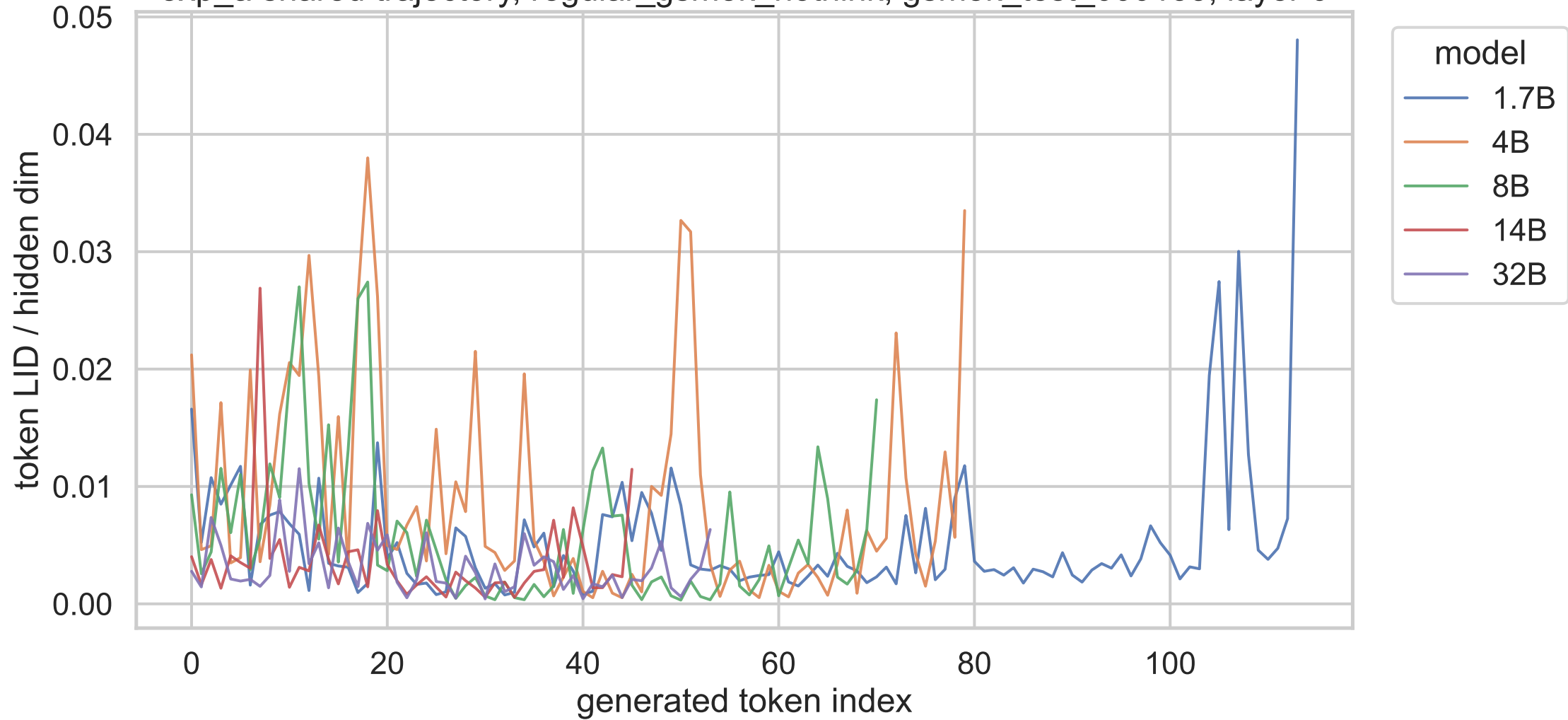
exp_a shared trajectory, regular_gsm8k_nothink, gsm8k_test_000153, layer 6
