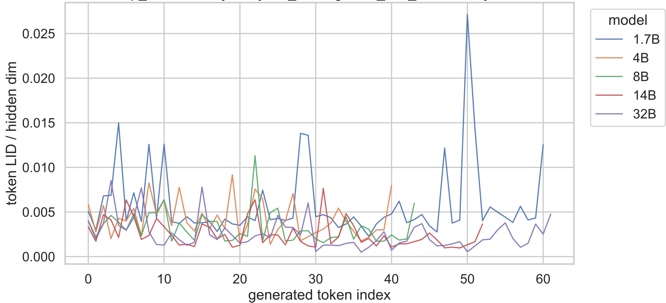
exp_c shared trajectory, no_think, gsm8k_test_000007, layer 13
