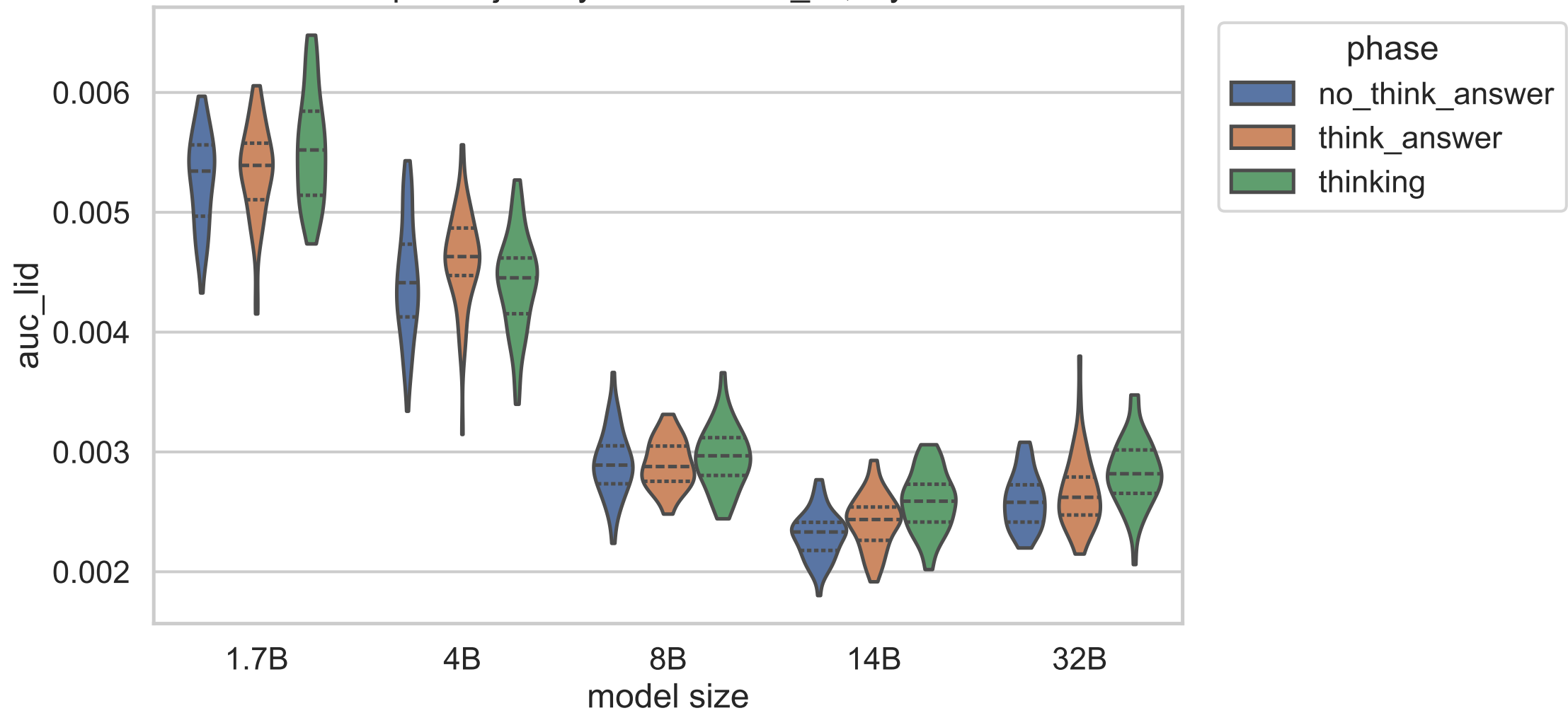
Exp C trajectory statistic: auc_lid, layer 13
