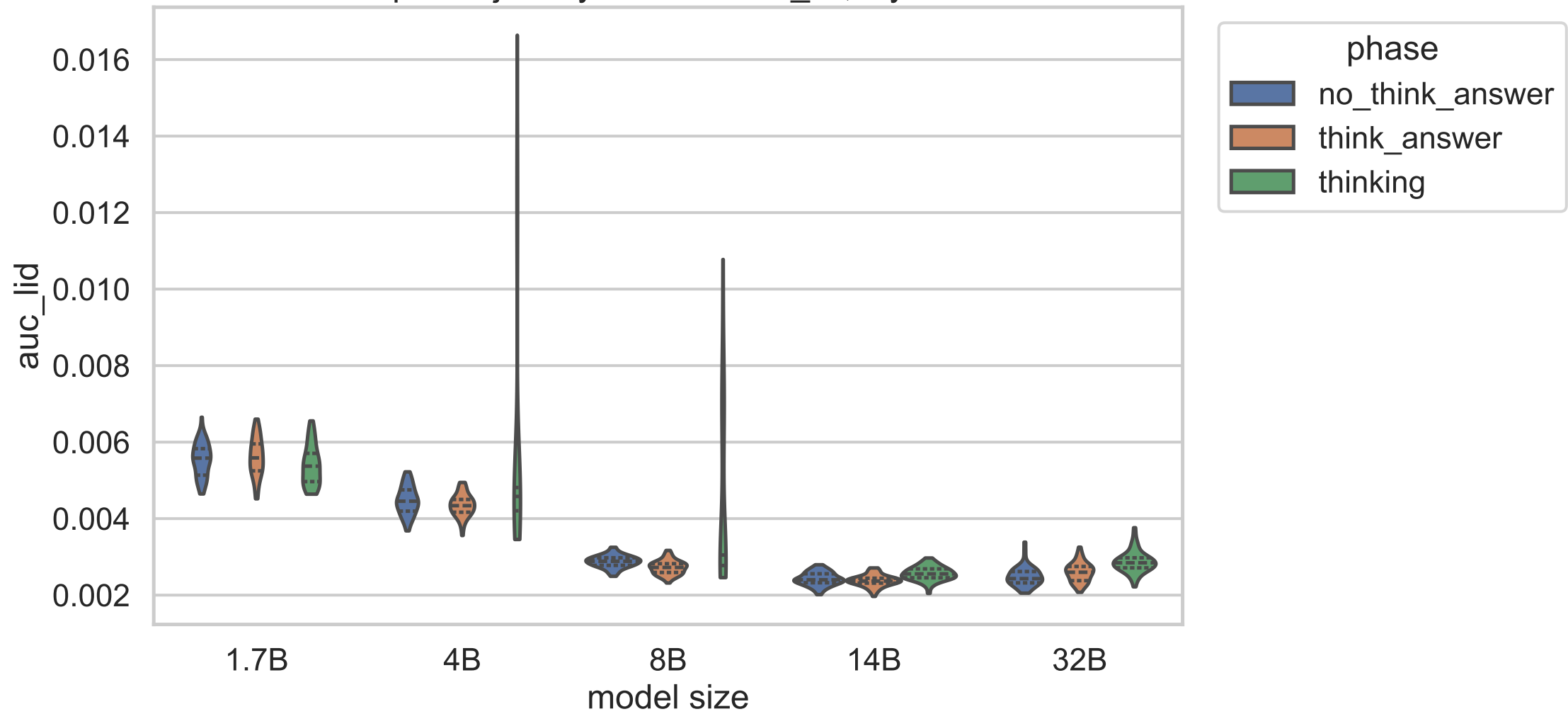
Exp C trajectory statistic: auc_lid, layer 20
