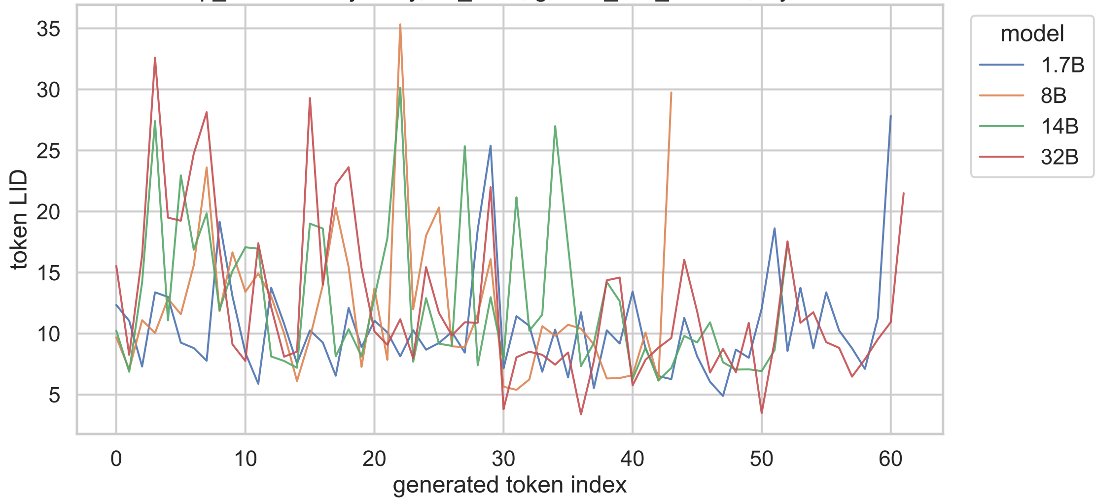
exp_c shared trajectory, no_think, gsm8k_test_000007, layer 20
