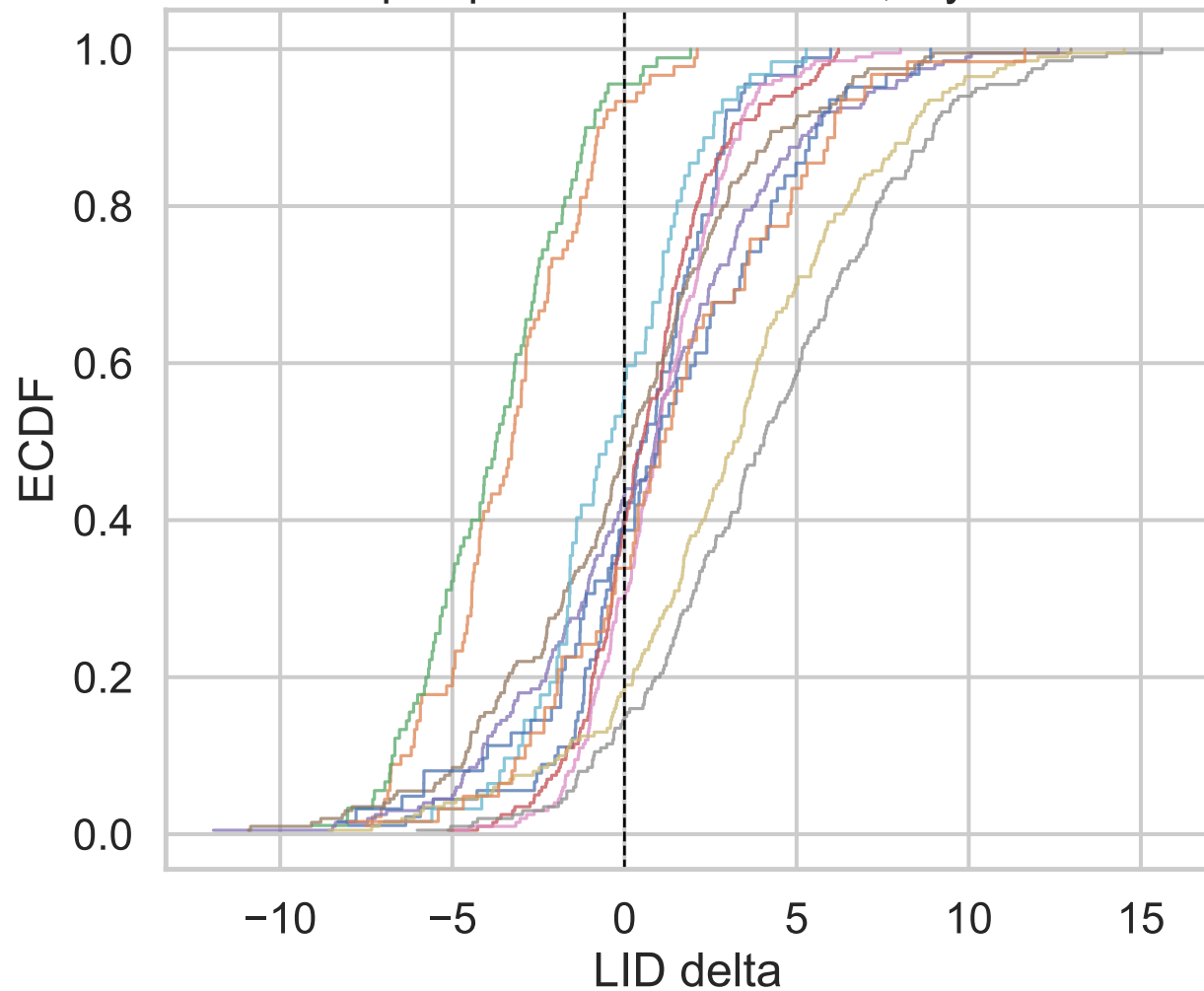
Exp C paired delta ECDFs, layer 6
