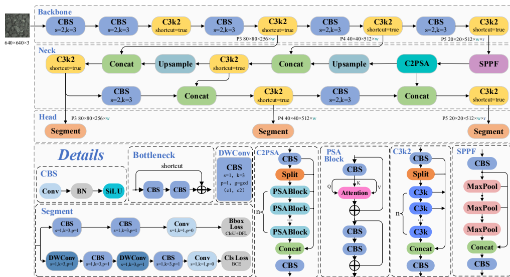
Gambar 2.5: Arsitektur YOLO11-seg
