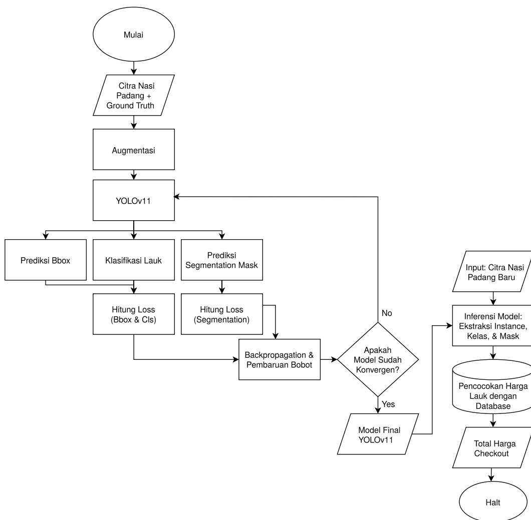
Gambar 2.3: Diagram alur pelatihan dan inferensi sistem checkout otomatis
