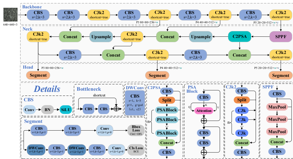
Gambar 2.4: Arsitektur YOLO11-seg
