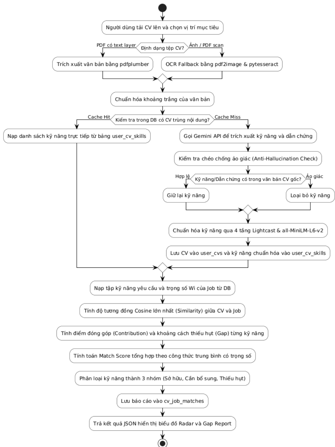
Hình 3.12: Sơ đồ luồng xử lý từ khi người dùng tải CV lên đến khi nhận kết quả so khớp.
