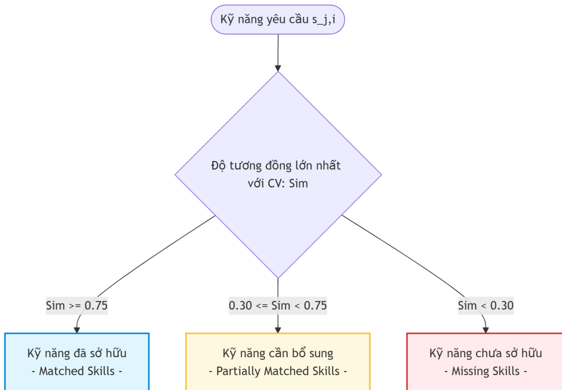
Hình 3.13: Quy tắc phân loại kỹ năng phục vụ báo cáo khoảng cách năng lực.
