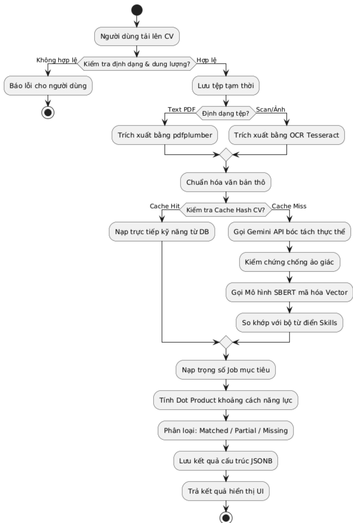
Hình 3.22: Sơ đồ luồng xử lý từ khi người dùng tải CV lên đến khi nhận kết quả so khớp.
