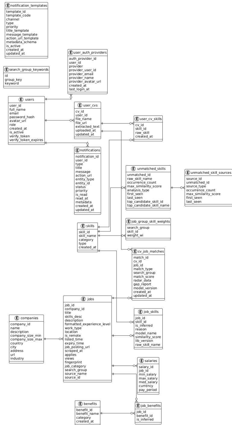
Hình 3.5: Sơ đồ mối quan hệ thực thể (ERD) của hệ thống.
