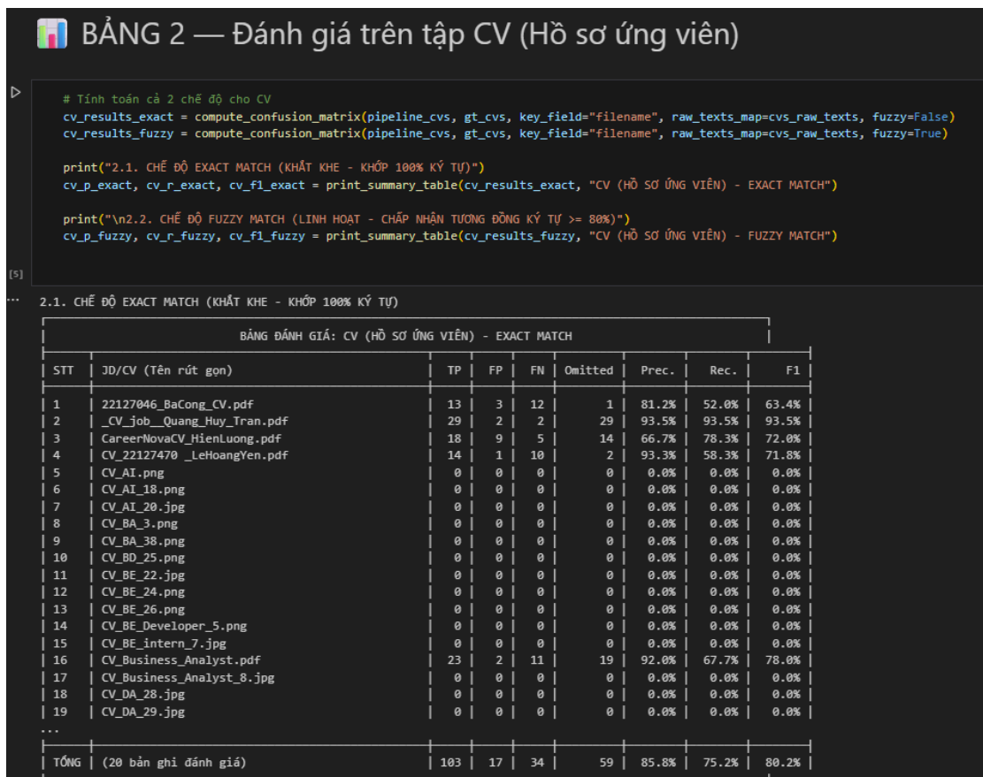
Hình 5.11: Bảng đối soát chi tiết TP/FP/FN của tập hồ sơ ứng viên (CV); hàng TỔNG đạt 103/17/34 (85,8%/75,2%/80,2%). Có thể thấy rõ 15 tệp CV dạng ảnh (.png/.jpg) cho kết quả 0 do OCR chưa đọc được nội dung.
