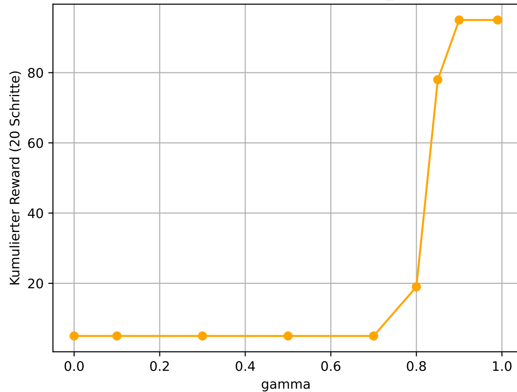
gamma vs. kumulierter Reward ab s_init=(0,4)
