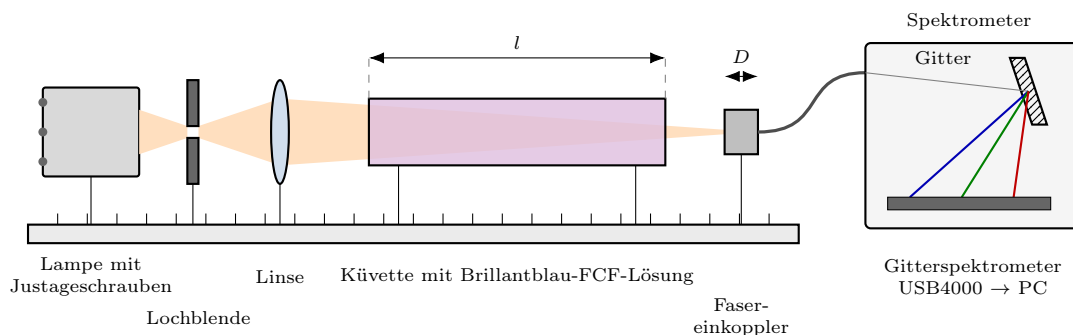
Abbildung 2: Aufbau (nicht maßstäblich). Die Küvette der Länge l verändert den Durchmesser D des Lochblendenbildes am Fasereinkoppler, siehe (9). Im Spektrometer zerlegt das Gitter das Licht auf die CCD-Zeile.
