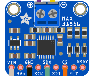
ADAFRUIT 3263 MAX31856
