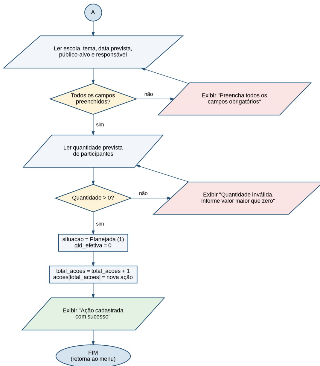
Figura 3 – Cadastro de ação (parte 2): demais campos, quantidade prevista e gravação. Fonte: elaborado pelos autores (2026).
