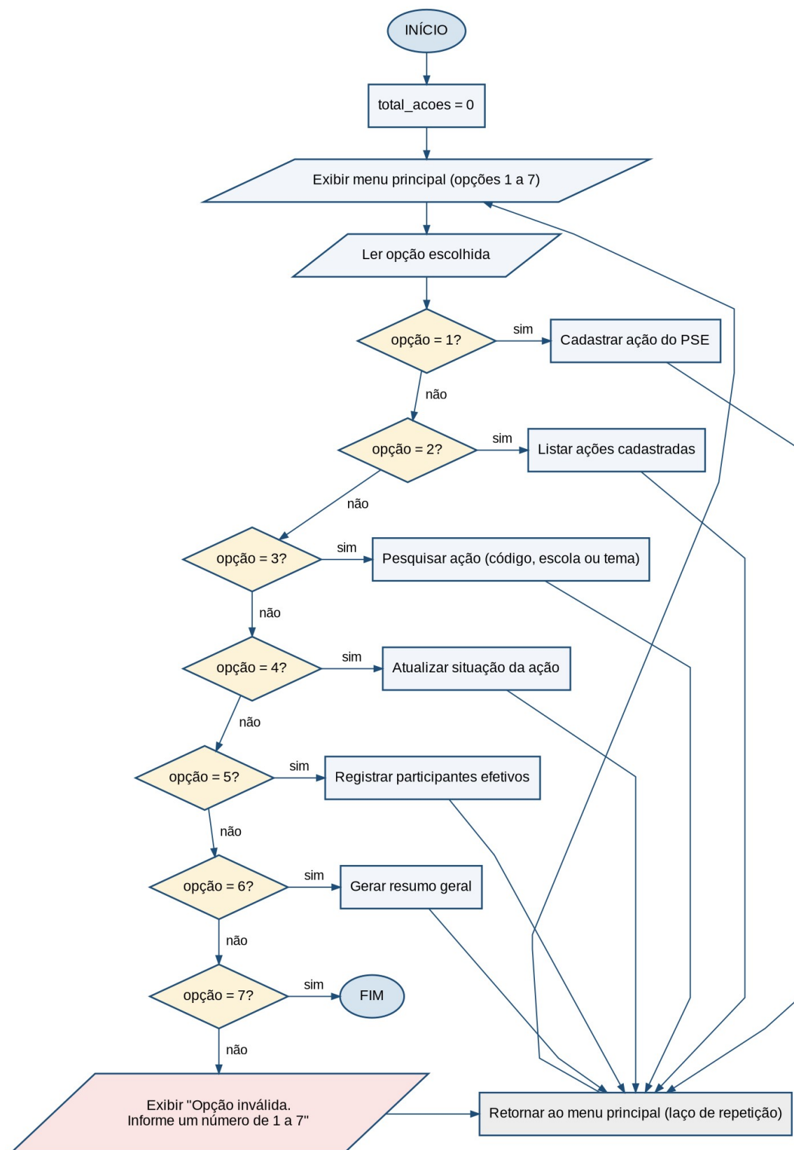
Figura 1 – Fluxograma geral do sistema PSE em Ação. Fonte: elaborado pelos autores (2026).
