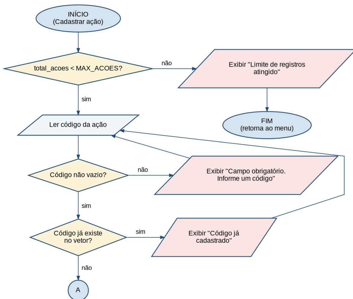
Figura 2 – Cadastro de ação (parte 1): limite de registros e validação do código. Fonte: elaborado pelos autores (2026).
