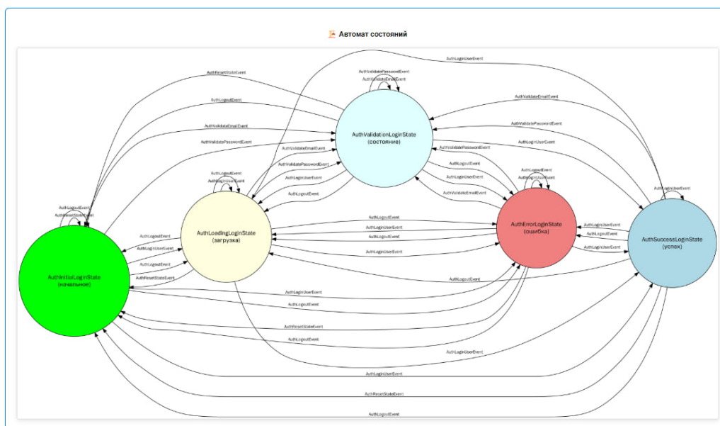
Рисунок 3 — Атомат состояний блока.
