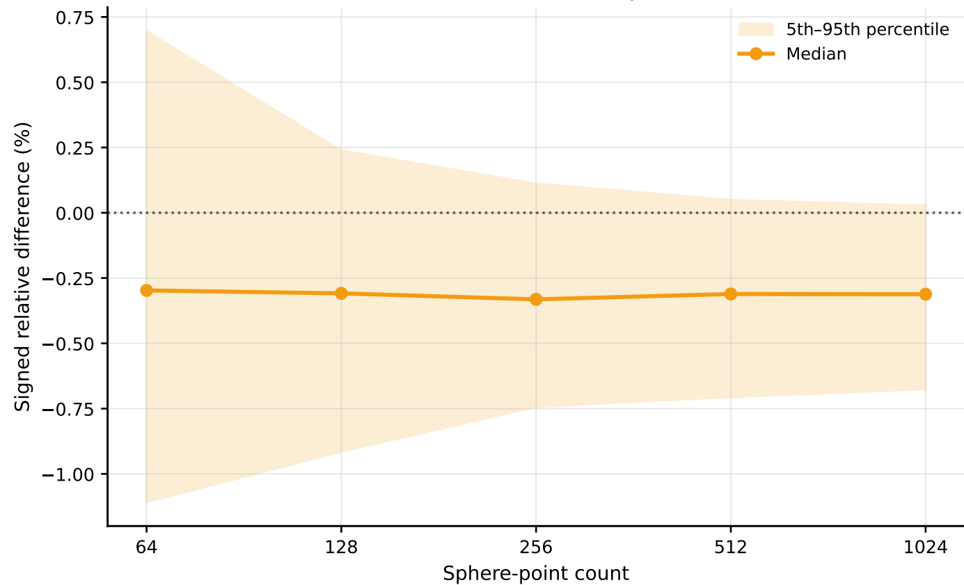
zsasa f64 vs MDTraj
