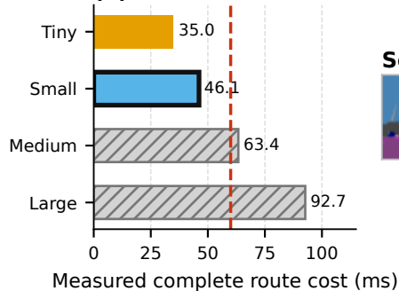
(d) E1 · Hailo-8 · B=60 ms
