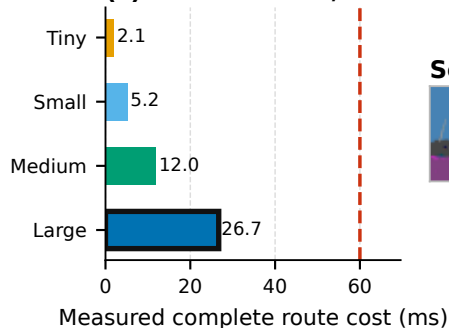
(c) E3 · TensorRT/CUDA · B=60 ms
