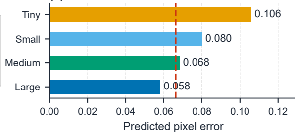
(e) E1 · Hailo-8 · medium/large infeasible · B=60 ms
