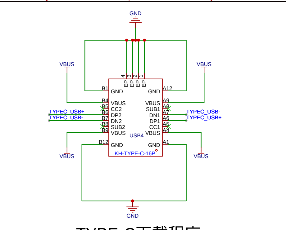
TYPE-C下载程序
