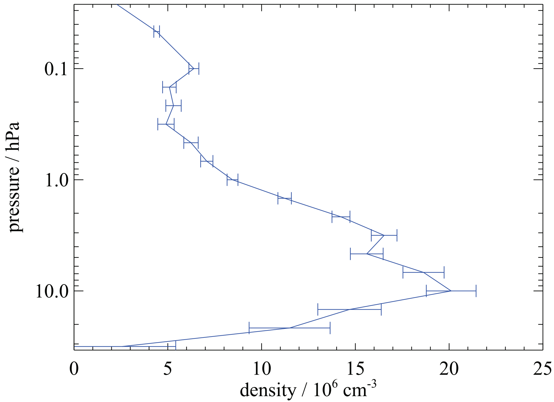
(f) HO2 v3
