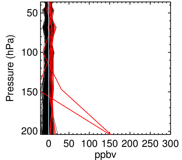
MLS SO2
