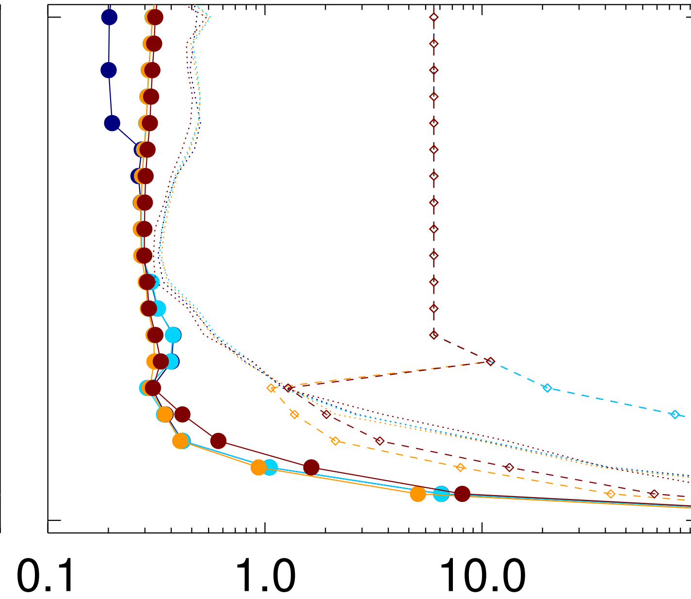
Precision
