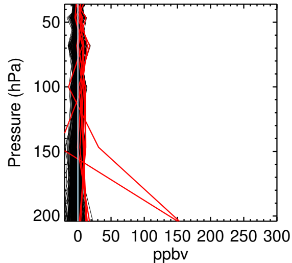
MLS SO2
