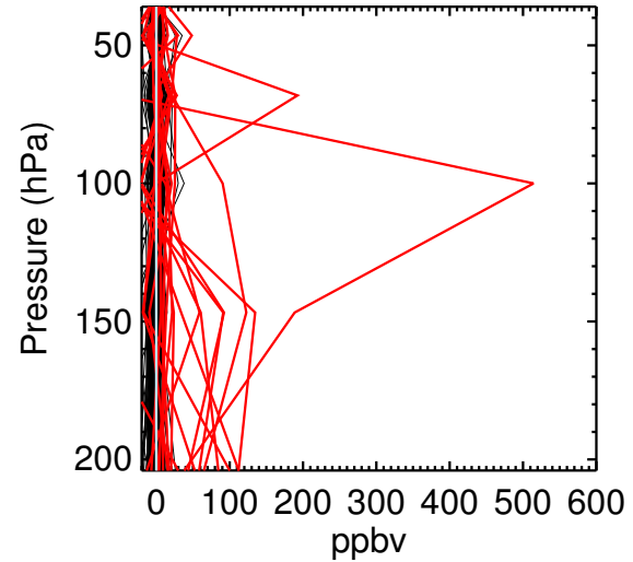
MLS SO2
