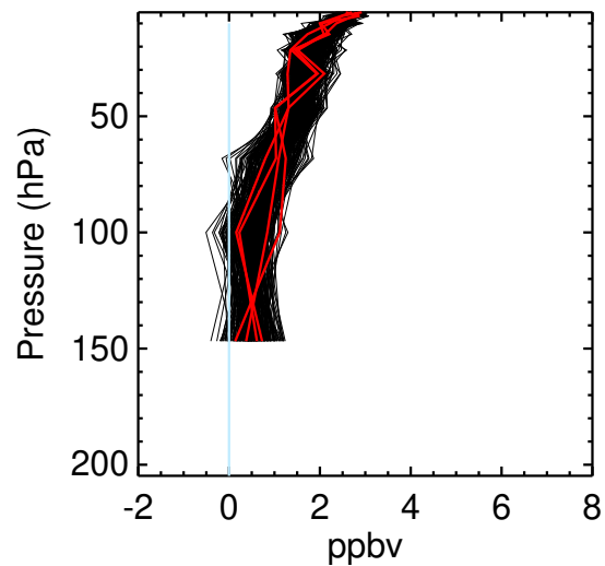
MLS HCI
