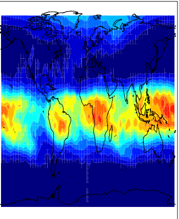
MLS V03.30
