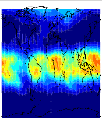
MLS V02.20
