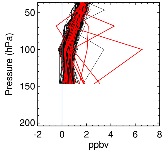
MLS HCI
