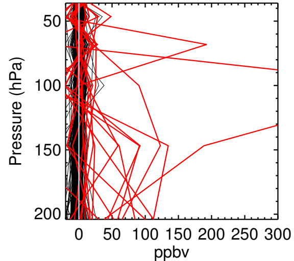
MLS SO2
