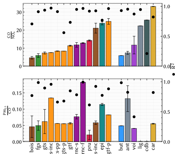
Figure 4. – Rapports globaux \frac{CO}{NO_x} et \frac{PM_{2,5}}{CO} , combustible végétaux (gauche) et fossiles (droite) ( R^2 superposés, p < 0,001 ).
