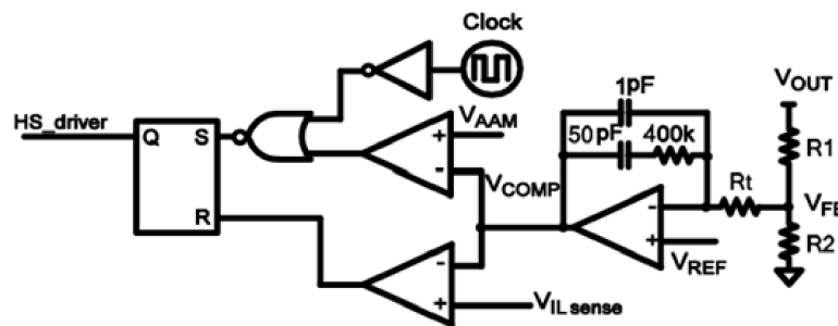
Figure 5.5.: Spannungswandler AAM-Regelbetrieb
