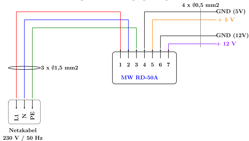
Figure 13.1.: Versorgungsschaltplan
