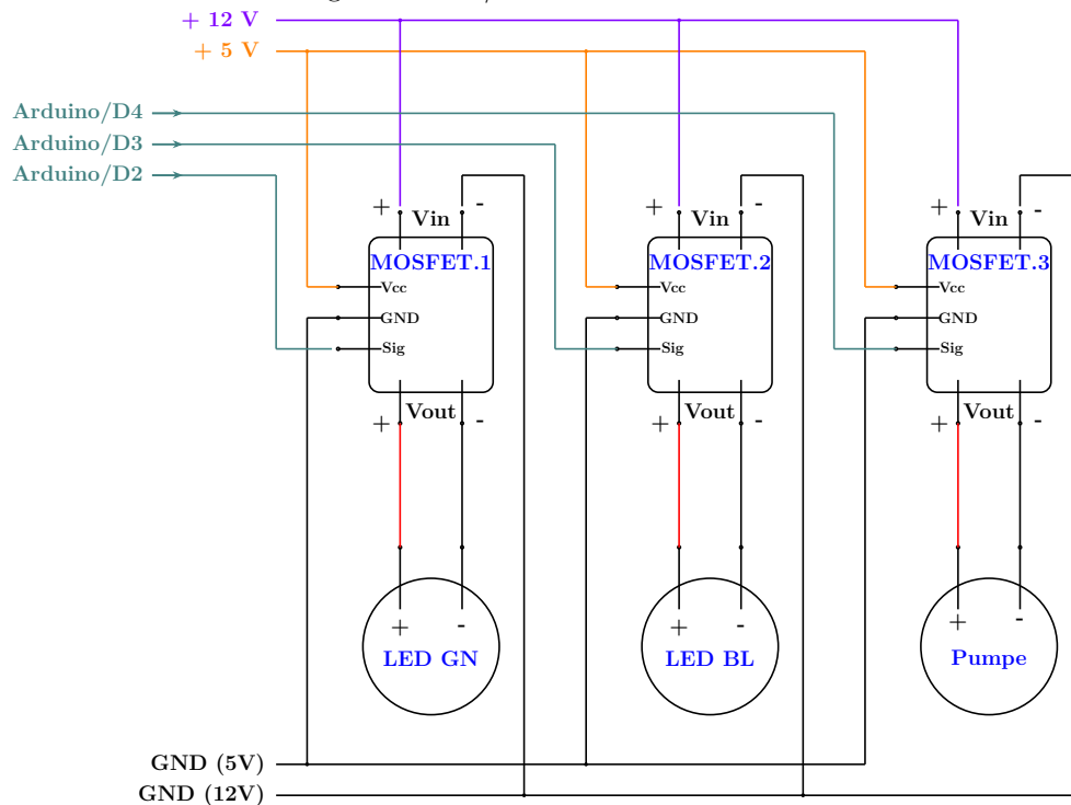
Figure 13.3.: 5/12 V Netz mit Aktoren
