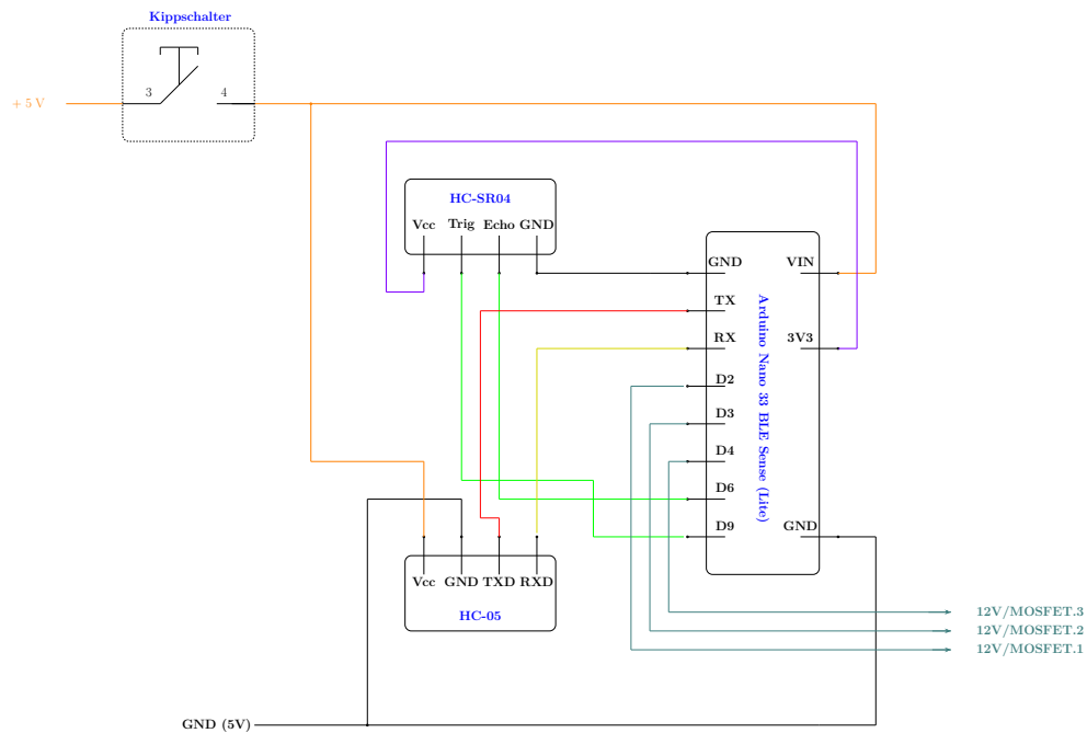
Figure 13.2.: Schaltplan: Arduino-basierte Steuerungseinheit mit Bluetooth-Kommunikation
