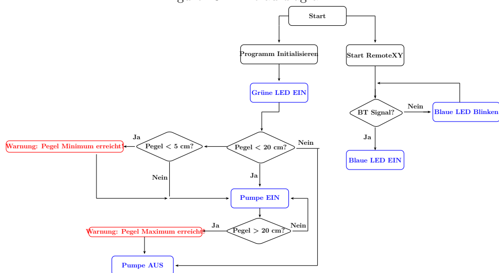
Figure 13.4.: Ablaufdiagramm
