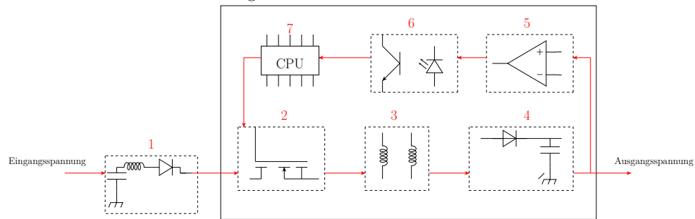
Abbildung 9.1.: Aufbau eines Schaltnetzteils
