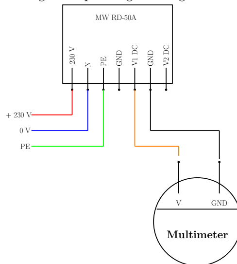
Abbildung 9.3.: Spannungsmessung des Netzteils
