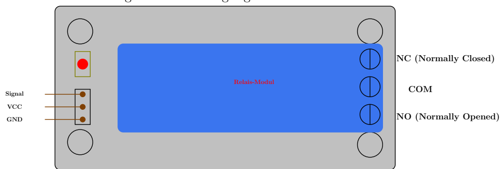
Abbildung 12.1.: Pin-Belegung und Aufbau des Relais-Moduls
