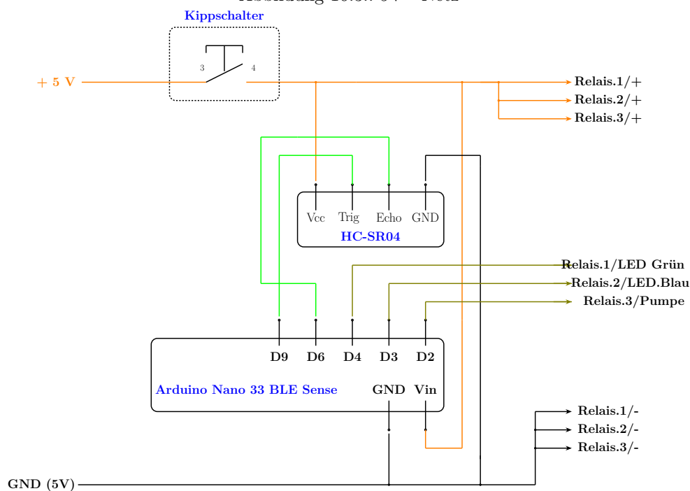
Abbildung 16.3.: 5V - Netz
