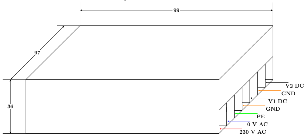
Abbildung 9.2.: Skizze des Netzteils
