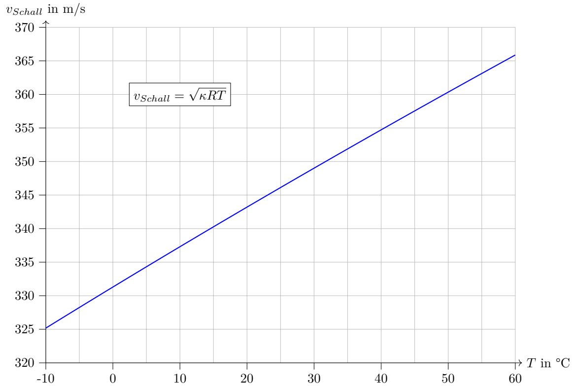
Abbildung 7.2.: Ausbreitungsgeschwindigkeit von Schall in Luft
