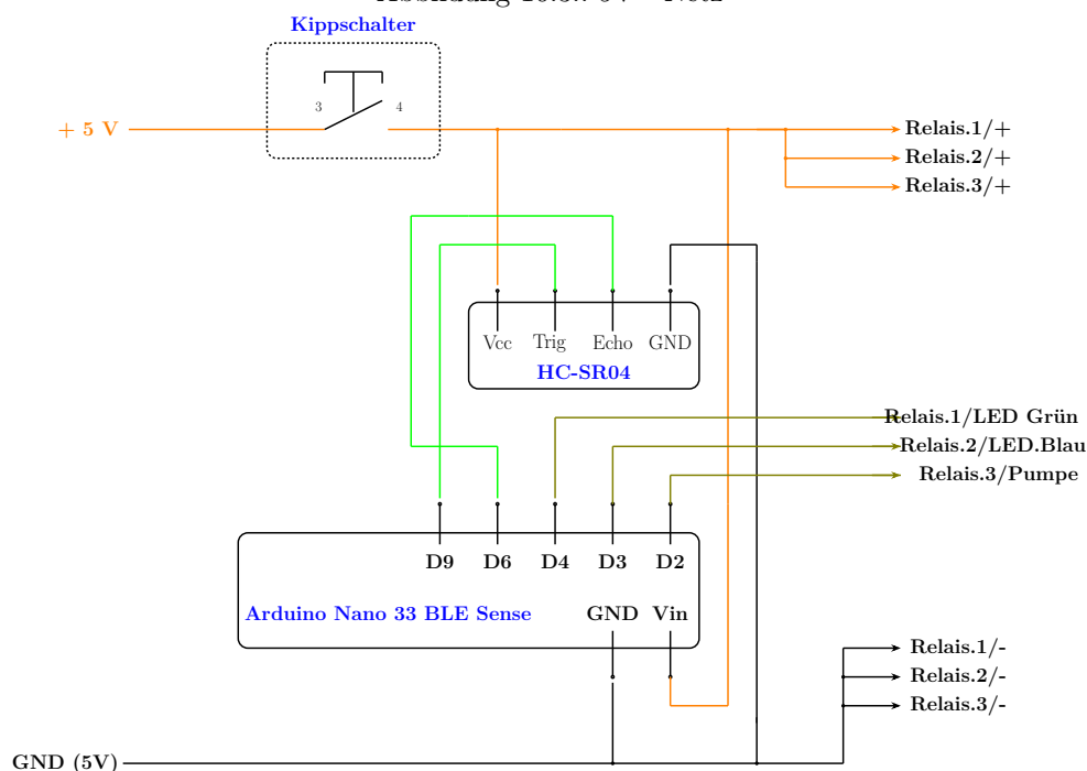
Abbildung 16.3.: 5V - Netz
