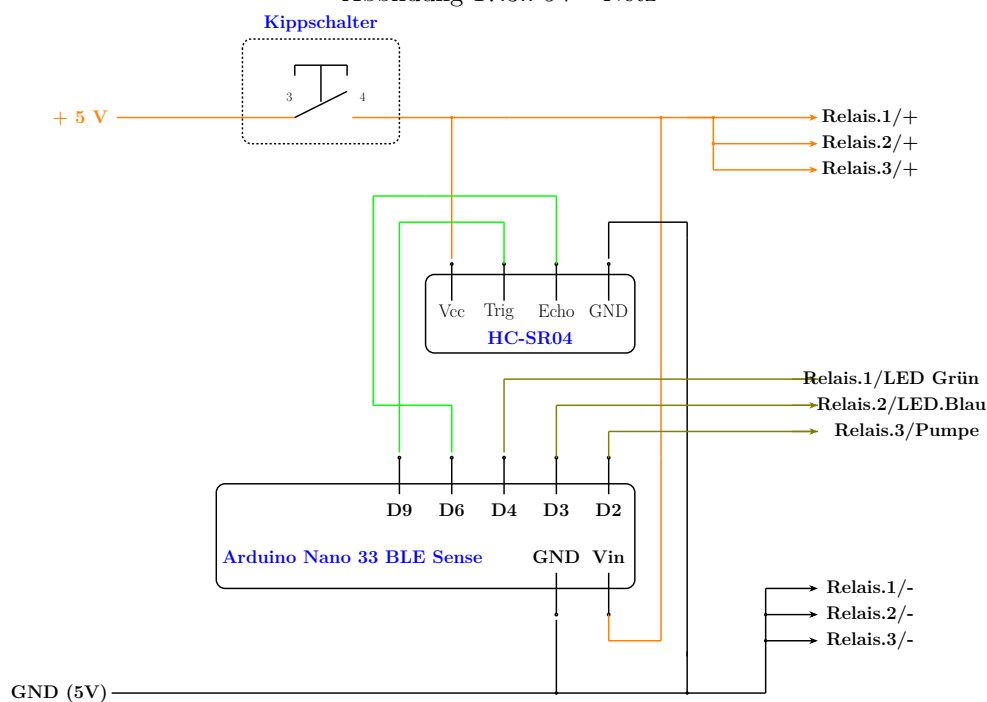
Abbildung 17.3.: 5V - Netz
