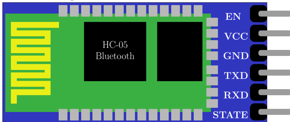
Figure 10.1.: Skizze des Bluetooth Moduls HC-05
