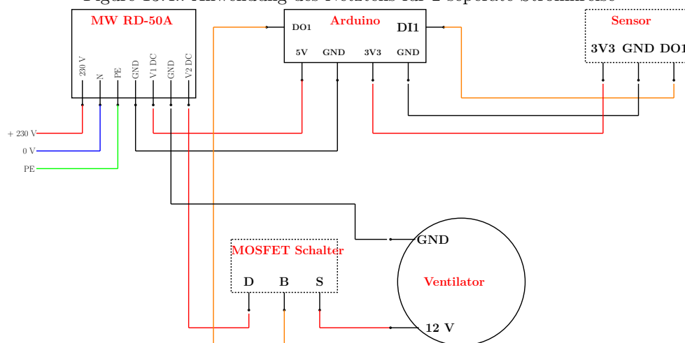
Figure 13.4.: Anwendung des Netzteils für 2 separate Stromkreise
