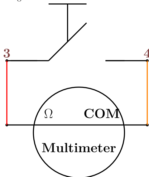
Figure 15.2.: Messen des Widerstands
