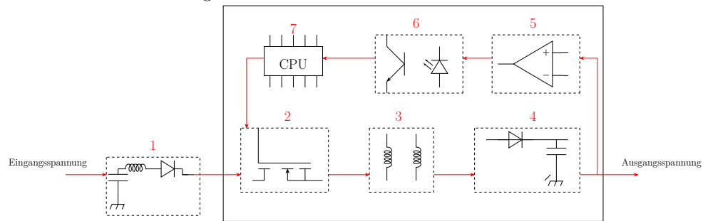
Figure 13.1.: Aufbau eines Schaltnetzteils
