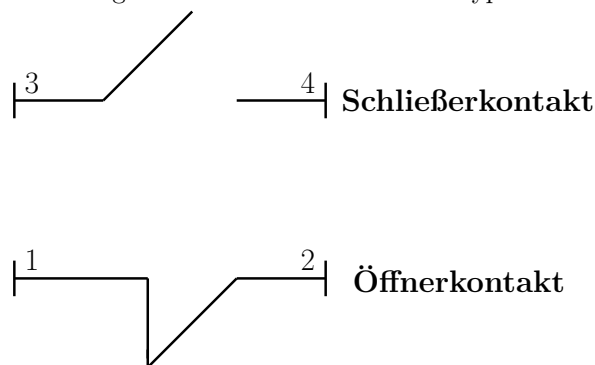
Figure 15.1.: Skizze der Schaltertypen
