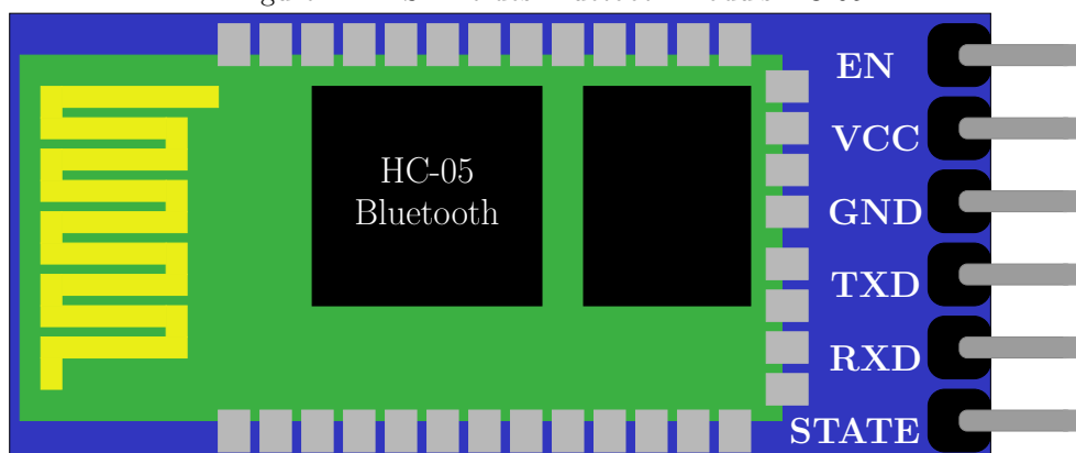
Figure 14.1.: Skizze des Bluetooth Moduls HC-05
