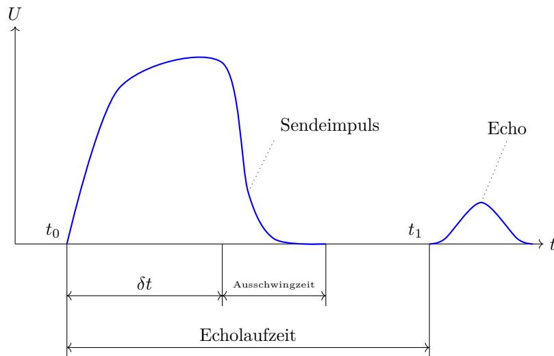
Figure 11.3.: Spannungsverlauf Schallwandler bei einer Echo-Laufzeit-Messung, nach [HS23]
