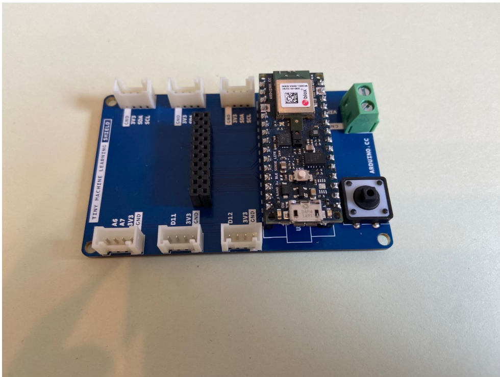
Figure 9.1.: Mikrocontroller gesteckt auf dem Shield
