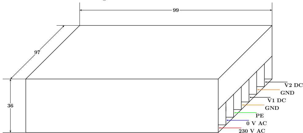
Figure 13.2.: Skizze des Netzteils
