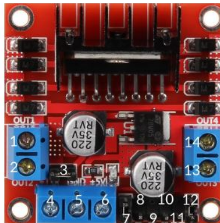
Figure 27.2.: Treiber mit Beschriftung
